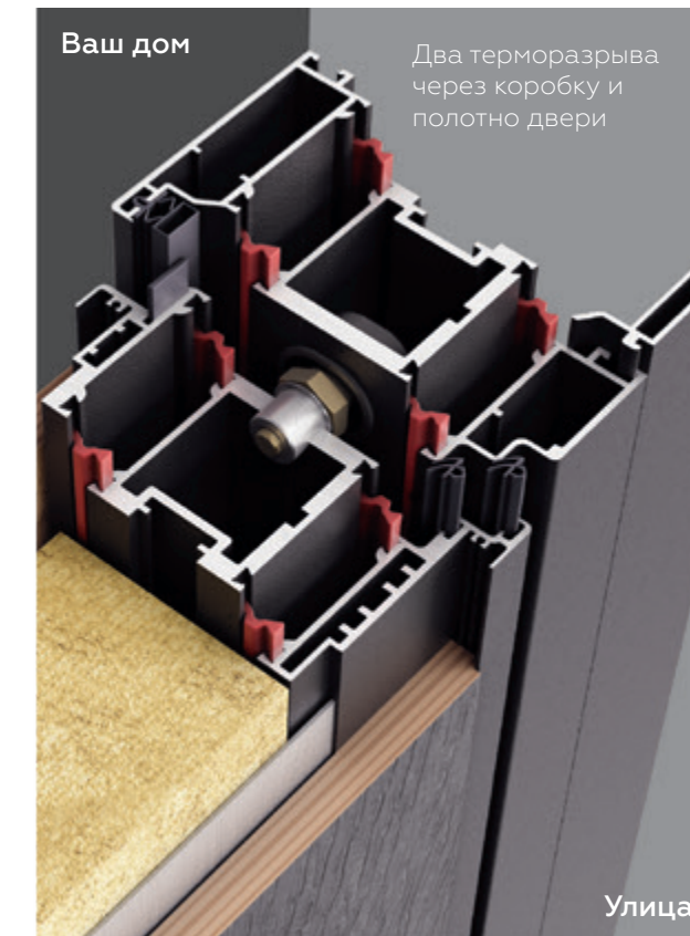
Два контура терморазрыва в алюминиевой двери
